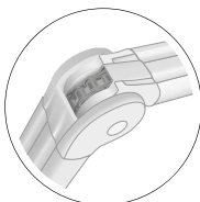
Bras à chaînes à rouleaux Testés à 60 000 cycles
